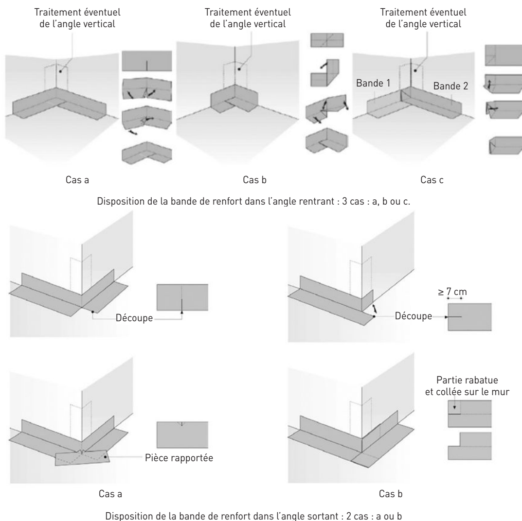
Figure 5 : pose des bandes de renfort des SPEC dans les angles
